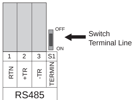
Fig. 16 - Blocchi morsetto collegamento seriale RS-485
