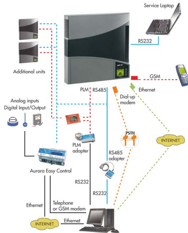
Fig.12 - Comunicazione dati a Aurora
