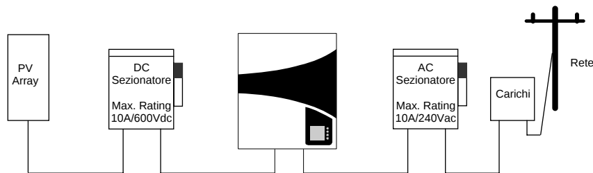
Fig.8 - Schema generico di connessione elettrica
