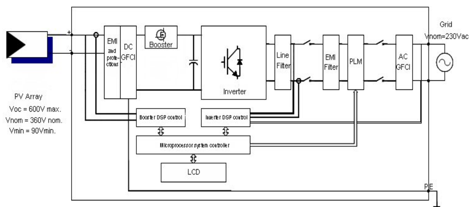
Fig.4 - Diagramma a blocchi AURORA
