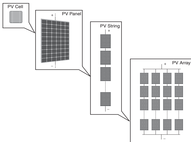
Fig.2 - Composizione Array
