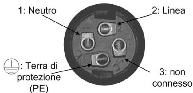
Fig. 11 - Connettore Binder
