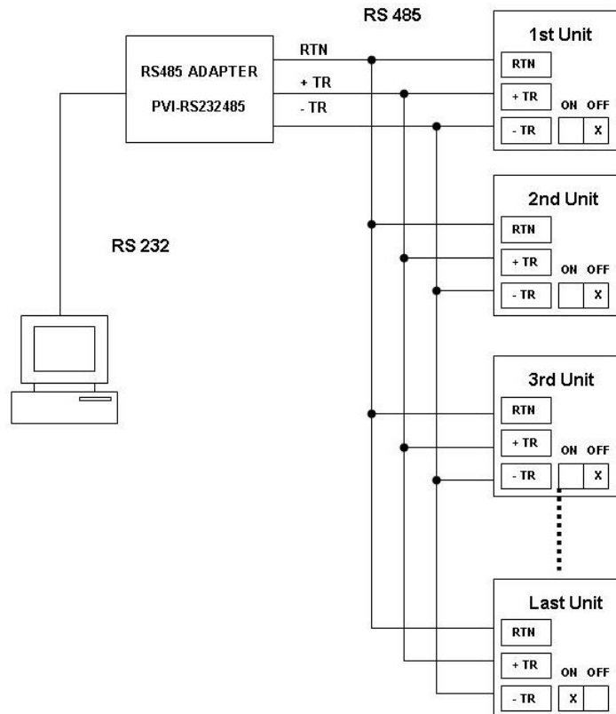
Fig.17 - Connessione multipla daisy-chain
