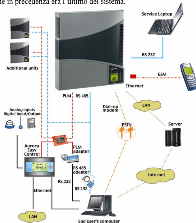
Fig.18 - Trasmissione dati all'AURORA Easy Control
